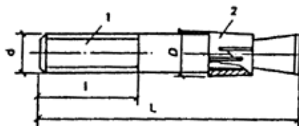
Рис. 1 прил. 1. Дюбель-шпилька распорная, тип 1 1 — распорная шпилька; 2 — разжимная цанга
