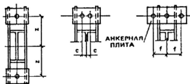
Рис.19. Схема расположения болтов для крепления стальных колонн решетчатого типа. Промышленный альпинизм, высотные работы http://www.moemstekla.ru 8 (903) 715-6540
