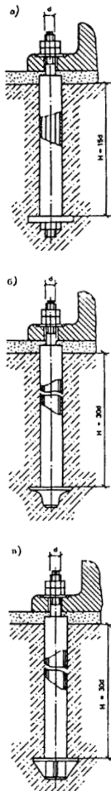
Рис. 2. Болты съемные, устанавливаемые после бетонирования фундаментов а — с плоской анкерной плитой (М12-М48); б — с литой анкерной плитой (М56-М125); в — со сварной анкерной плитой (М56-М100) Болты изогнутые, устанавливаемые в колодцах, приведены на рис 3.
