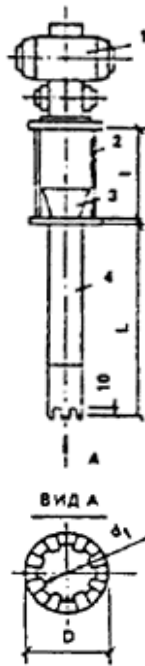
Рисунок прил. 5. Уплотнительное устройство 1 — вибратор; 2 — удлинитель; 3 — воронка; 4 — уплотнитель; L — выполняется по максимальной высоте болта на объекте
